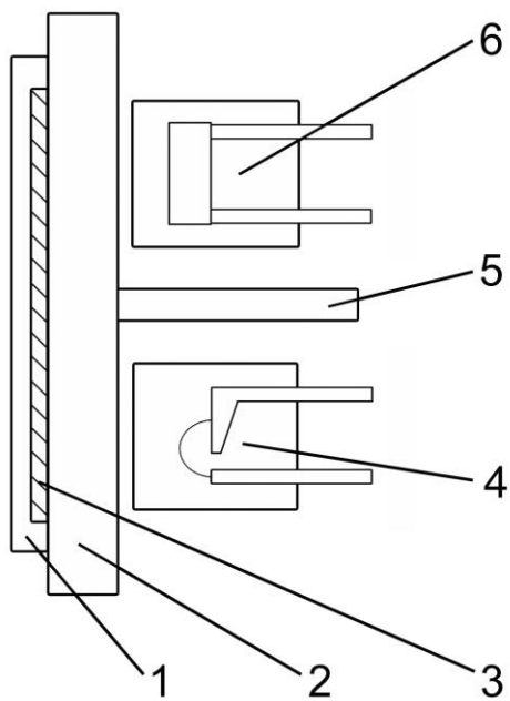
Detektor składający się z elementu aktywnego (1-3) (transparentne podłoże (2), warstwa europu (3) przykryta warstwą palladu (1)), źródła światła (4), nietransparentnej przegrody (5) oraz fotodetektora (6)
